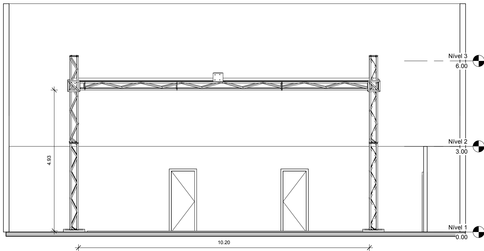
1 VISTA FRONTAL 1 : 50
