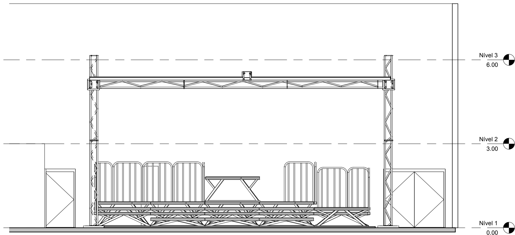
1 VISTA PLATEIA 1 : 50
